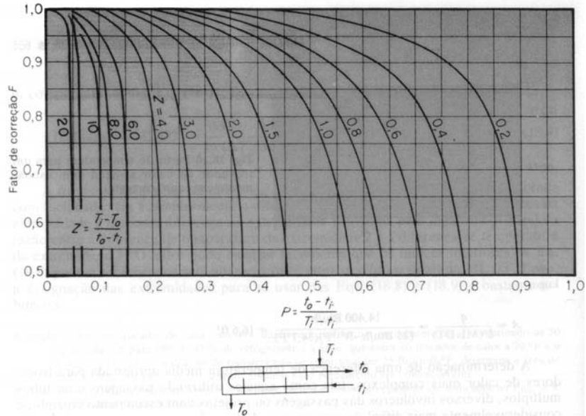
Fatores de correção para trocadores de calor com invólucro de uma passagem e duas passagens de tubos (ou múltiplos de dois).
